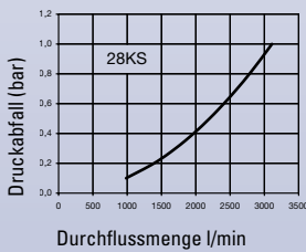
Durchfluss-Diagramm Luft
