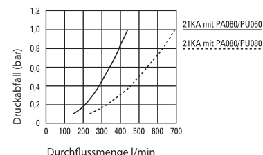
Durchflussdiagramme
