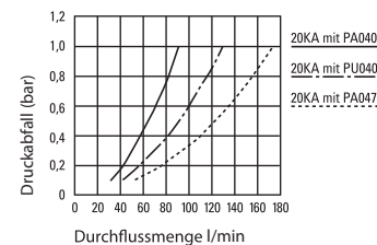
Durchflussdiagramme
